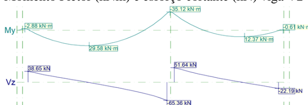
Figura 5 – Momento Fletor (kNm) e esforço cortante (kN) viga V2 – Cypecad.
