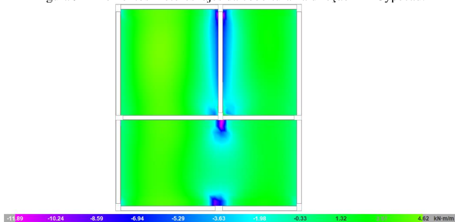
Figura 9 – Momentos Fletores lajes da cobertura na direção X – Cypecad.
