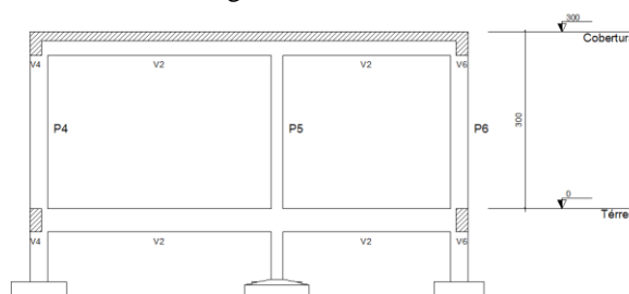
Figura 4 – Corte B-B
