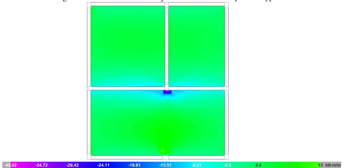
Figura 10 – Momentos Fletores lajes da cobertura na direção Y – Cypecad
