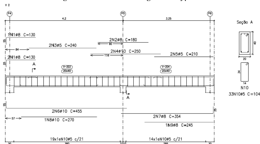
Figura 7 – Detalhamento viga V2 – Cypecad.
