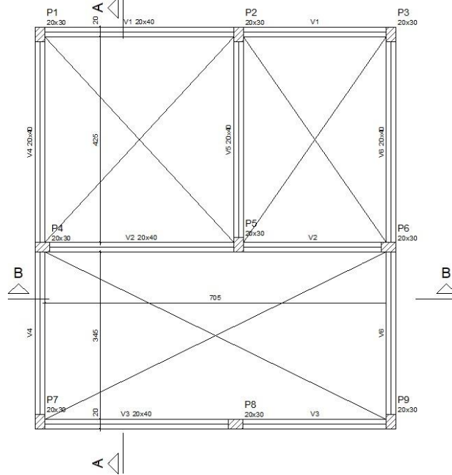
Figura 1 – Planta de forma do pavimento térreo
