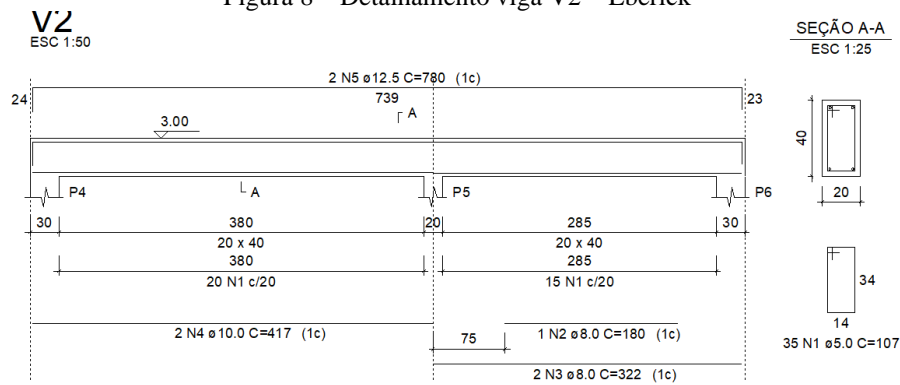
Figura 8 – Detalhamento viga V2 – Eberick
