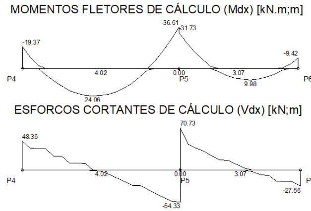
Figura 6 – Momento Fletor (kNm) e esforço cortante (kN) viga V2 – Eberick
