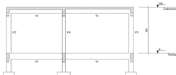
Figura 3 – Corte A-A
