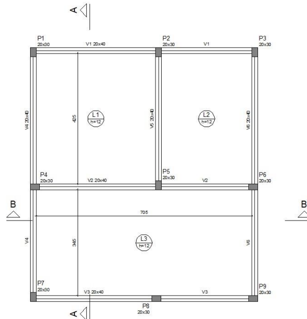
Figura 2 – Planta de forma da cobertura
