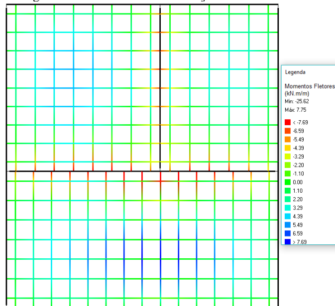
Figura 11 – Momentos Fletores lajes cobertura – Eberick.
