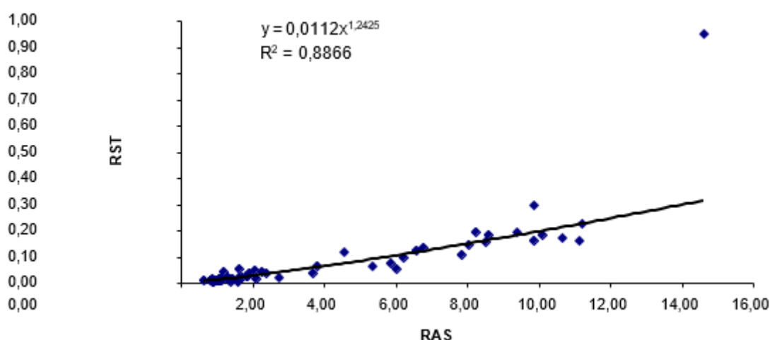
Figura 05: Variação da Relação de Sódio Trocável (RST) com a Relação de Adsorção de Sódio do solo (RAS).
