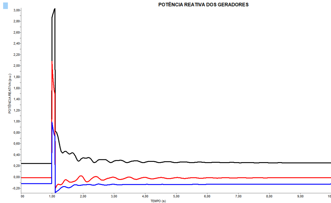
Figura 12: Potência Reativa pós-falta dos Geradores.
