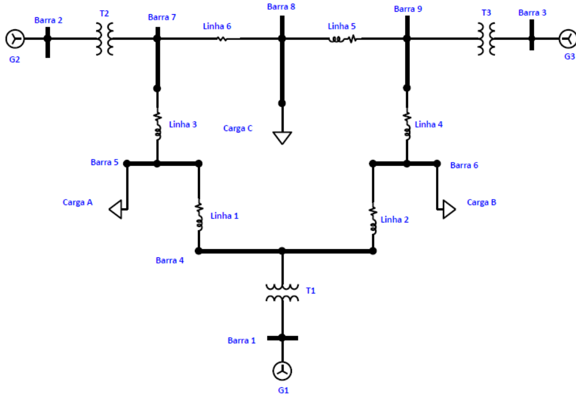
Figura 2: Circuito exemplo IEEE de 9 Barras.
