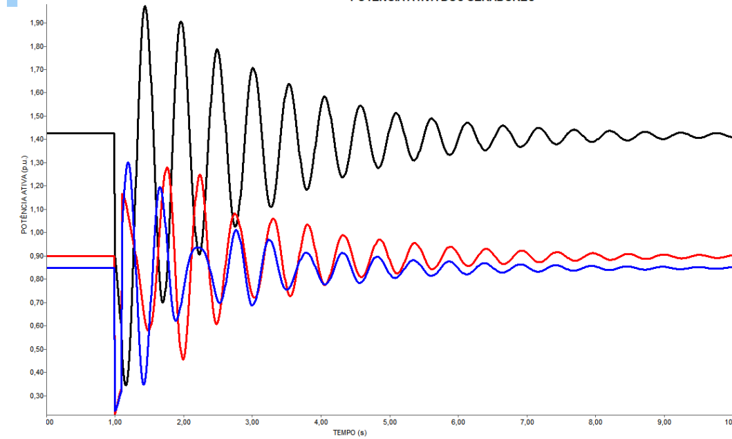
Figura 11: Potência Ativa pós-falta dos Geradores. POTÊNCIA ATIVA DOS GERADORES
