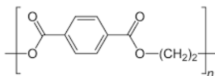
Figura 1. Estrutura química do PET.
