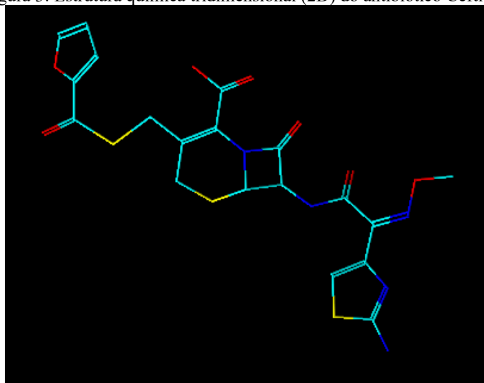
Figura 3: Estrutura química tridimensional (2D) do antibiótico Ceftiofur
