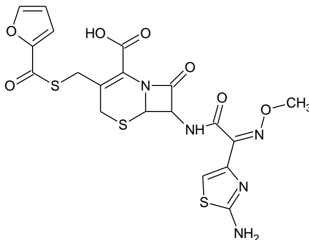
Figura 2: Estrutura química bidimensional (2D) do antibiótico Ceftiofur
